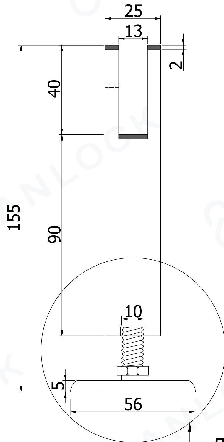
Фасад
