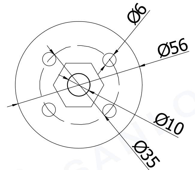
Деталь 1
