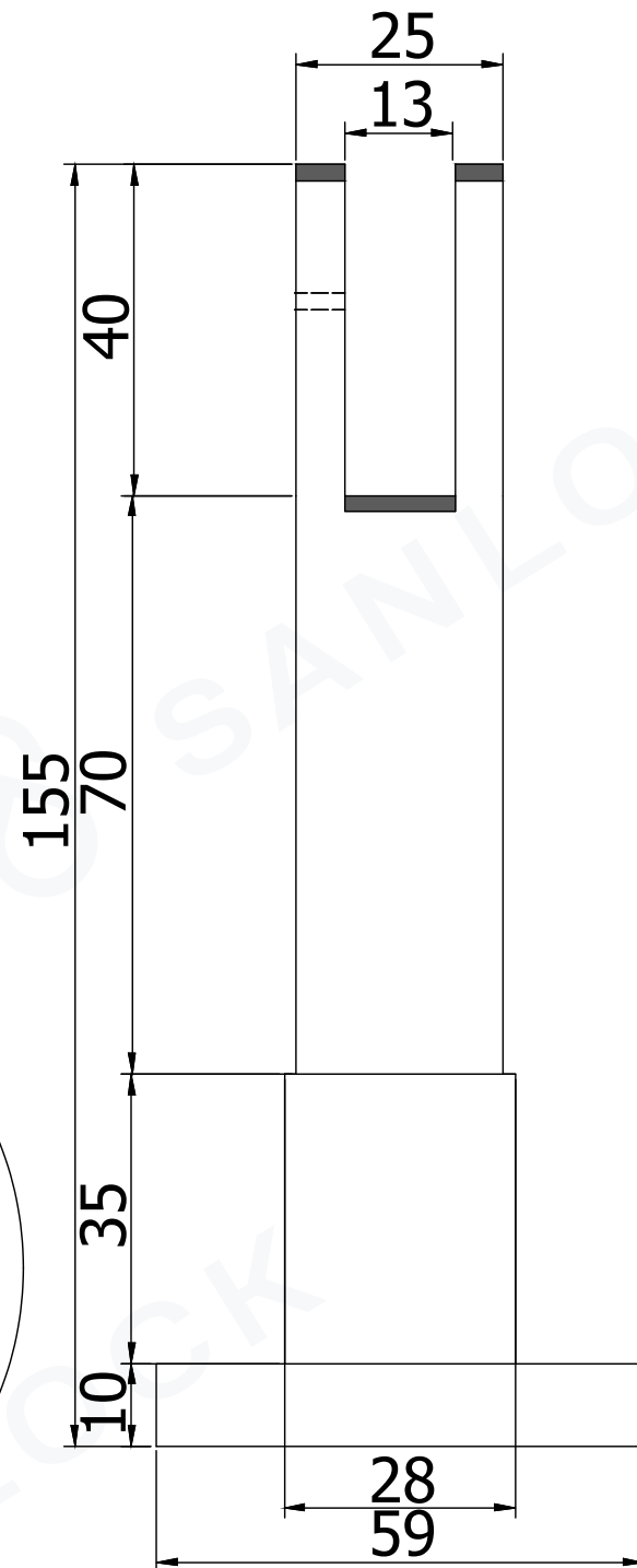
Фасад (в собранном виде)
